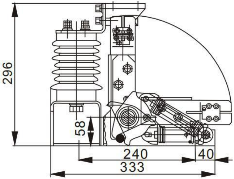
A-A
